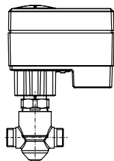
AME 13SU + + VZ D_y 15-20, VZL D_y 15-20
