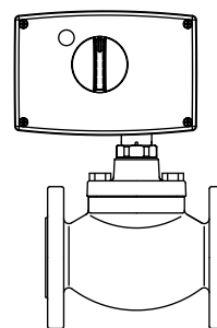
AME 23SU + + VB2 D_y 15-50
