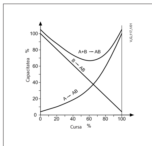
Caracteristici log./lin. vană (3 căi)
