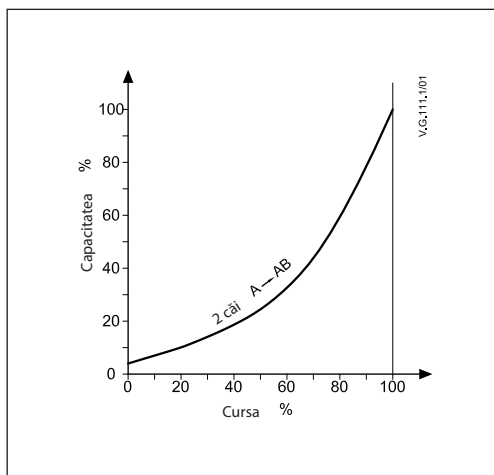
Caracteristici log. vană (2 căi)
