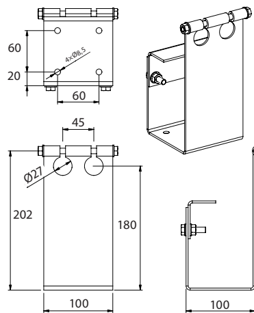
XB04, 24 laikiklis
