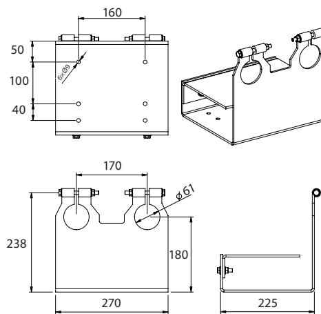
XB51 laikiklis
