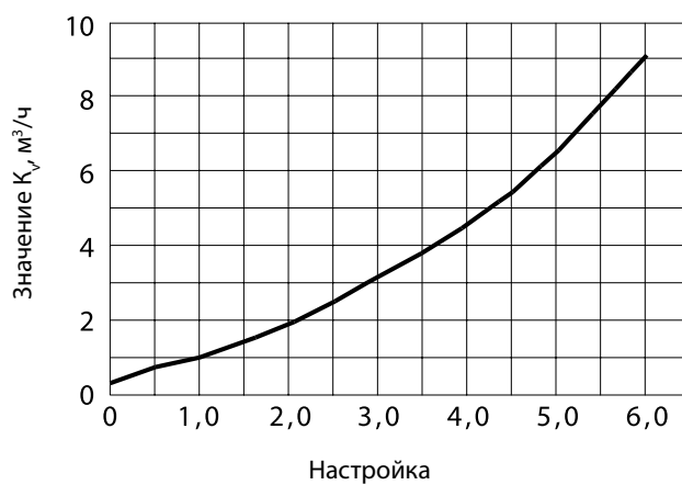
Расходная характеристика
