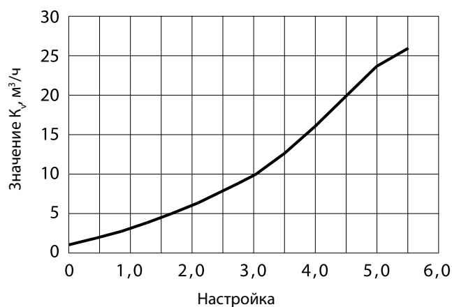
Расходная характеристика
