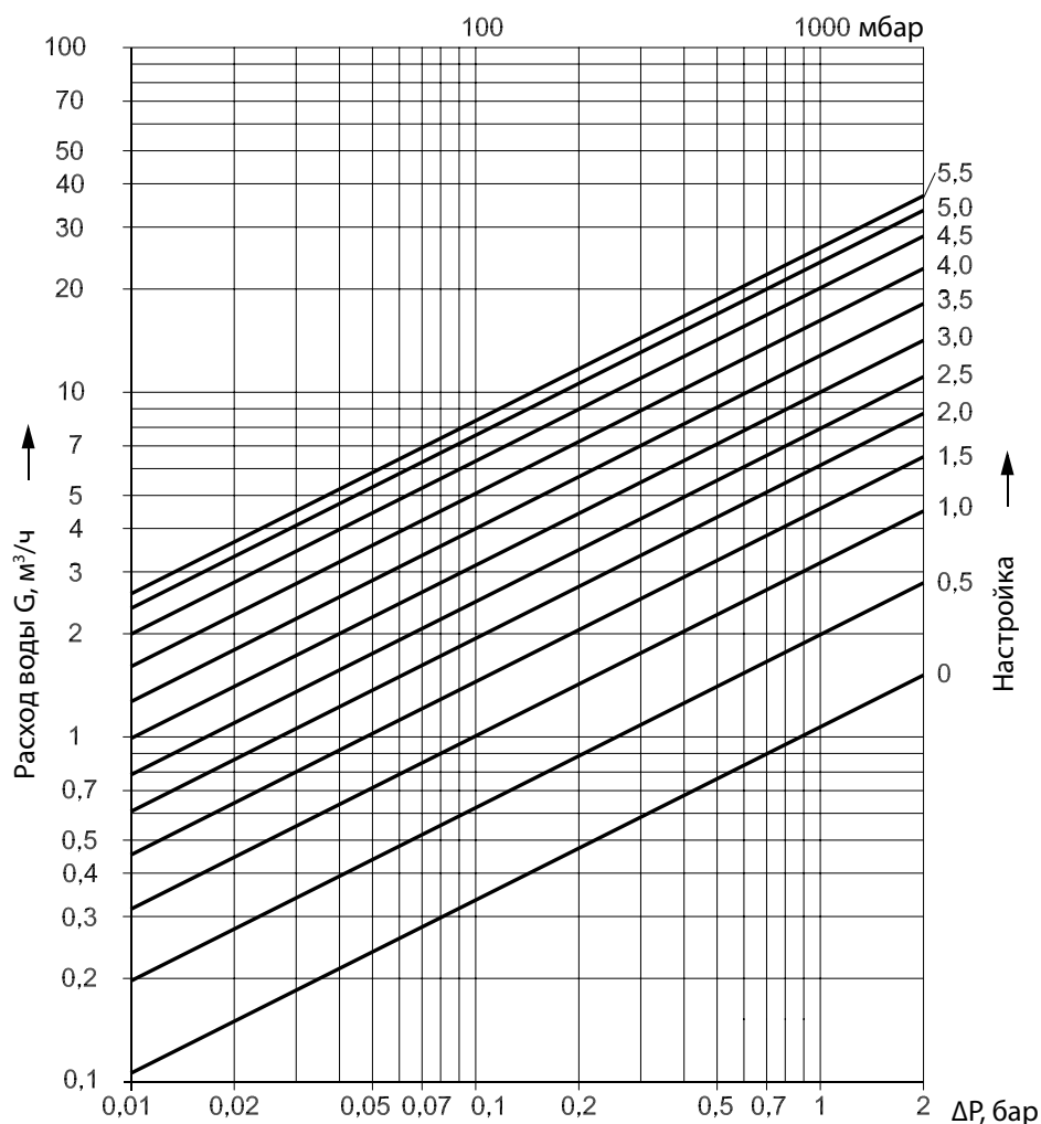
Диаграмма для настройки клапана Leno™ MSV-BD D_v = 40 мм
