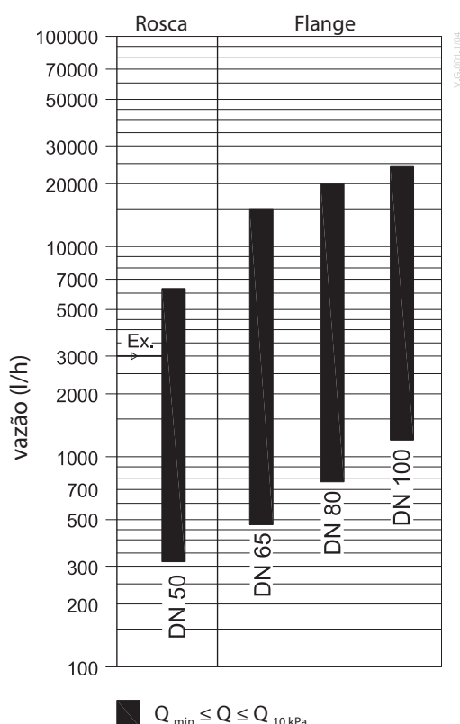
Fig. 7 Diagrama de coluna para o dimensionamento de válvulas ASV em \Delta p_v = 10 \text{ kPa} . Para valores de \Delta p_v diferentes, use o diagrama A do Apêndice.
