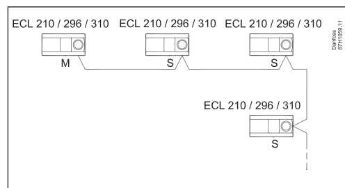
Підключення "керуючий/керований"
