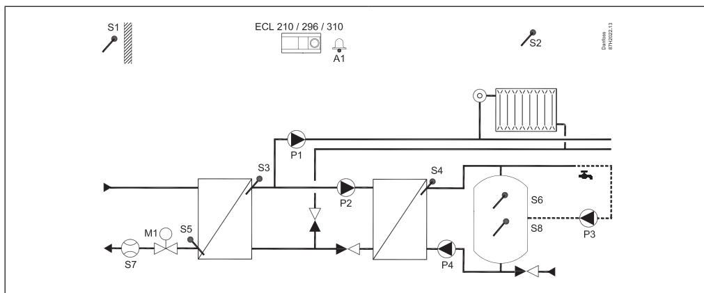
A247.1, приклад А: Система опалення з незалежною схемою приєднання та система заряджання накопичувального бака ГВП. Режим паралельної роботи або пріоритет ГВП
