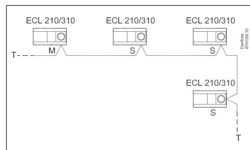
Master/slave připojení
