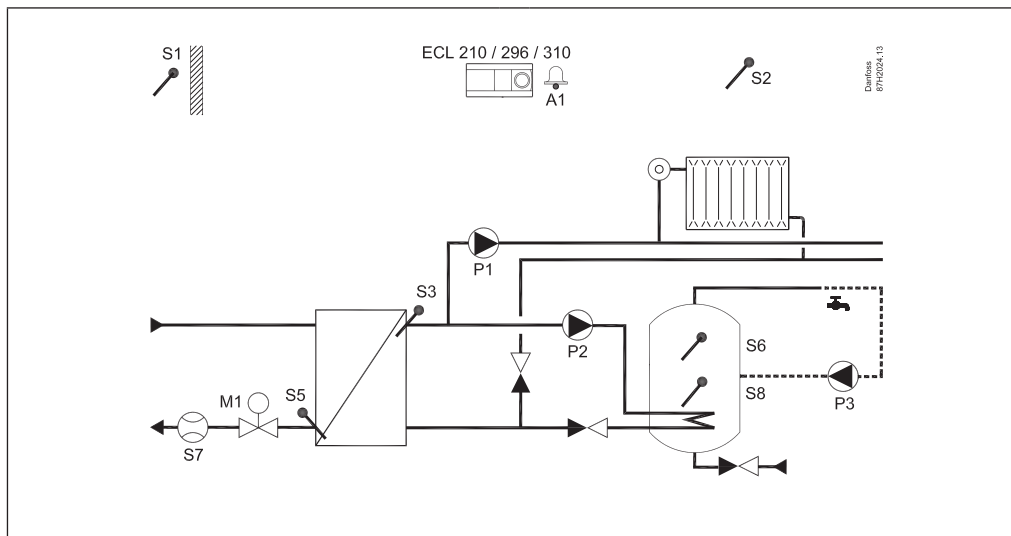
A237.2, пр. а: Индиректно свързана система за зареждане за отопление и БГВ
