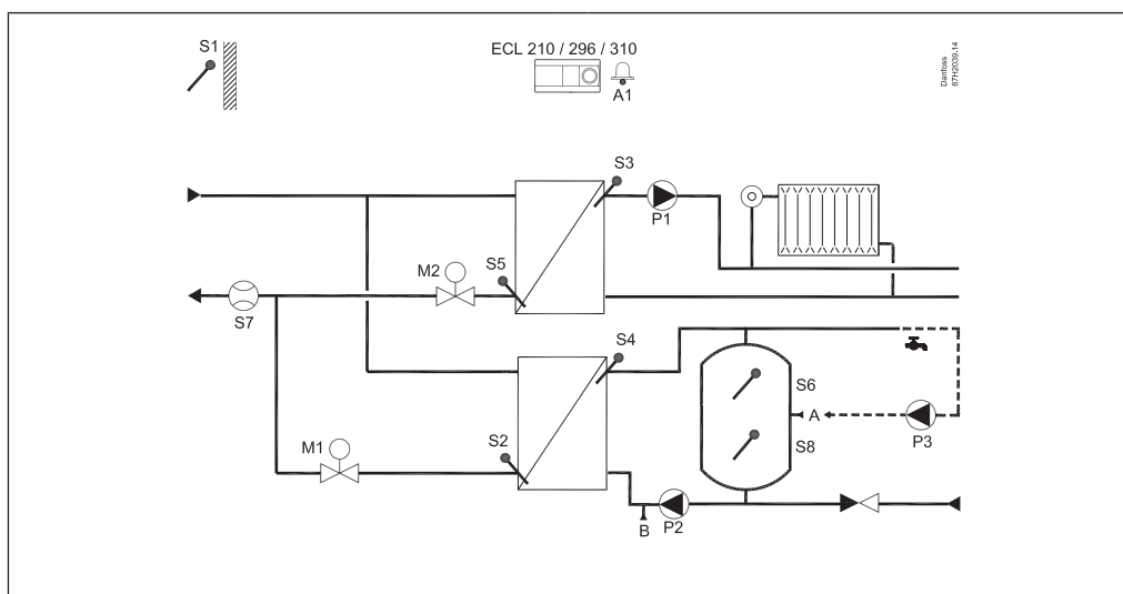
A247.1, пр. а: Индиректно свързана система за зареждане на резервоари за отопление и БГВ Паралелен режим или приоритет на БГВ
