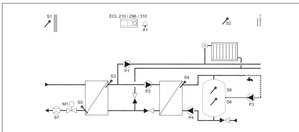
A247.1, пр. а: Индиректно свързана система за зареждане на резервоари за отопление и БГВ Паралелен режим или приоритет на БГВ
