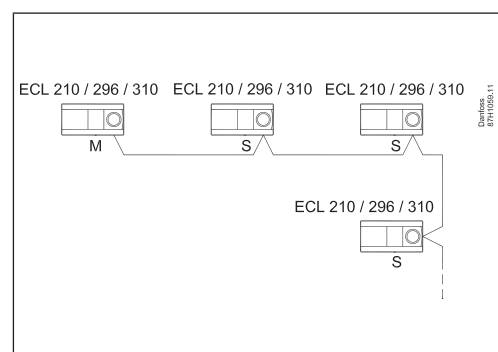
Връзки главен-подчинен
