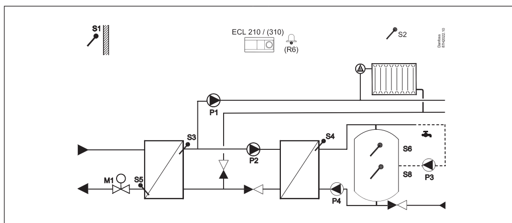
A247.1, пр. а: Индиректно свързана система за зареждане на резервоари за отопление и БГВ Паралелен режим или приоритет на БГВ
