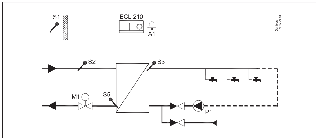
A217.3, пр. с: БГВ, отопление при поискване (ключ за поток) Със или без циркулация
