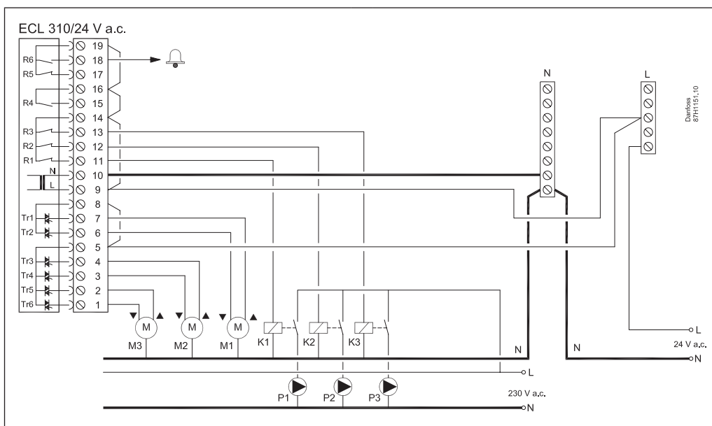
Пример за схема на свързване на ECL Comfort 310
