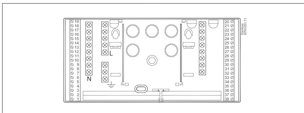
Основа на ECL Comfort 310 (може да се използва и за ECL Comfort 210).
