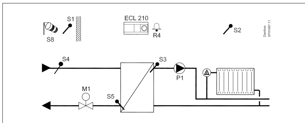
A230.1, пр. а: Индиректно свързана отоплителна система. Компенсация на вятъра като опция
