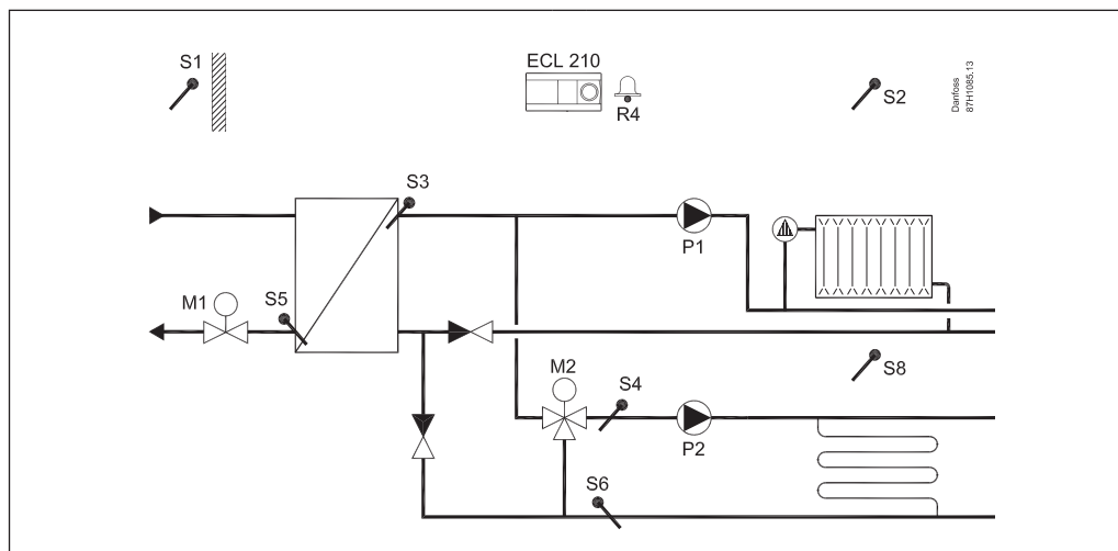
A260.1, пр. d: Две отоплителни системи. Контур 2 е подконтур на контур 1
