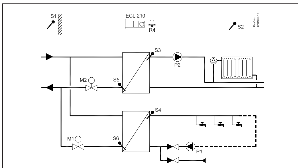
A266.1, пр. а: Отоплителна система и система за директно отопление с БГВ Паралелен режим или приоритет на БГВ
