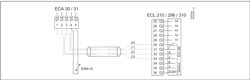
Схема на свързване на ECL Comfort 310/310B и ECA 30/31
