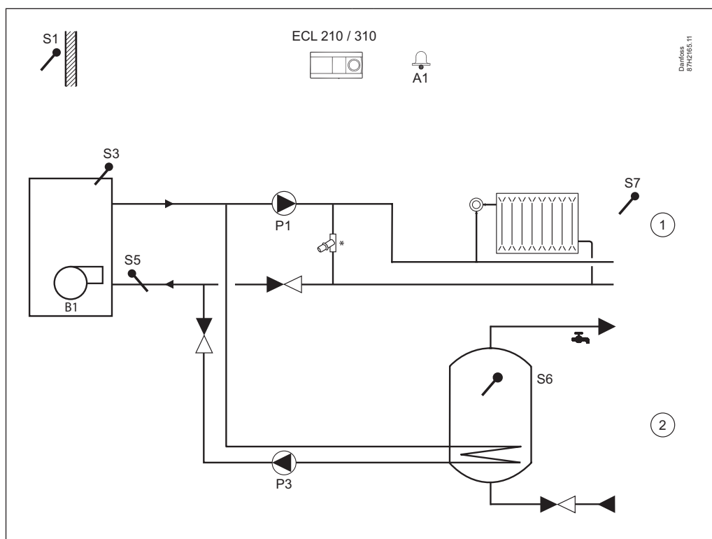
A275.2, eks. a: Varmeanlæg med 1-trins-kedel og varmtvandsbeholder
