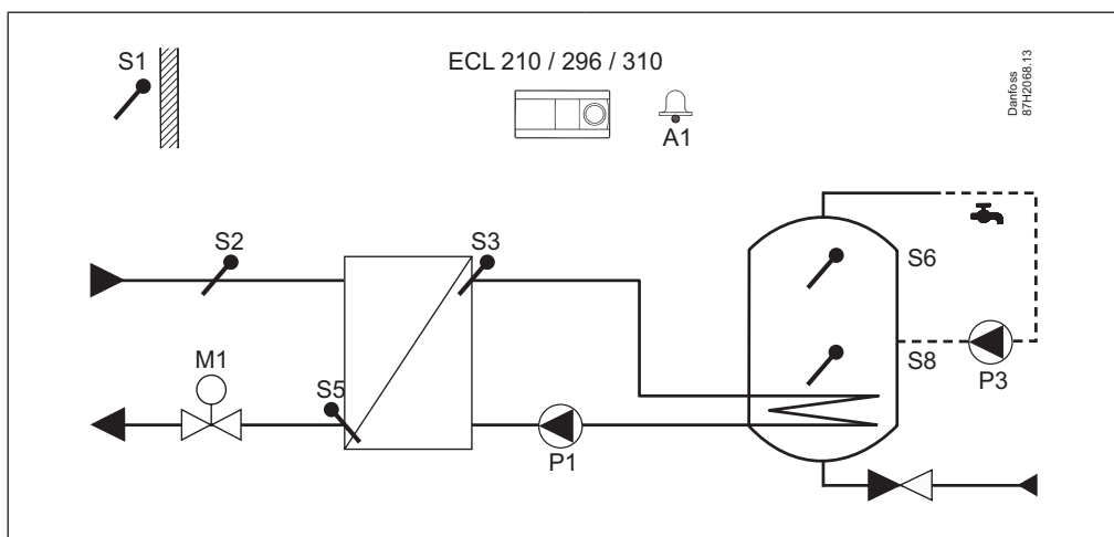
A217.2, Bsp. a: WW-Speicherladesystem mit Vorregelkreis
