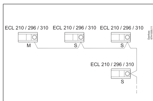
Anschlüsse für Haupt- und Folgeregler
