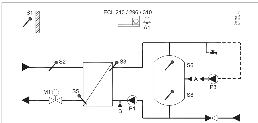
A217.1, Bsp. b: WW-Speicher mit innenliegender Heizschlange
