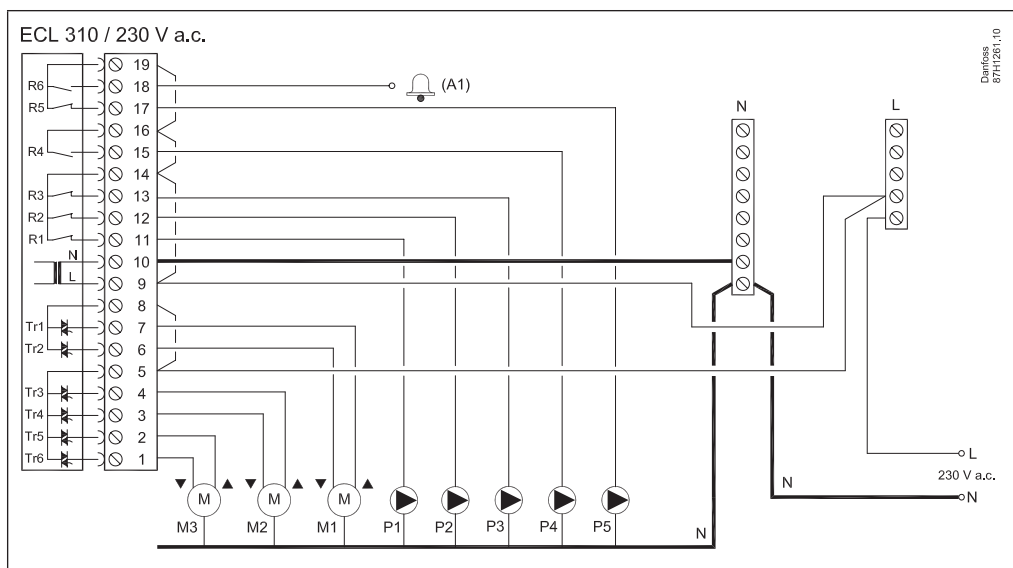
Esimerkki ECL Comfort 310 -johdotuksesta
