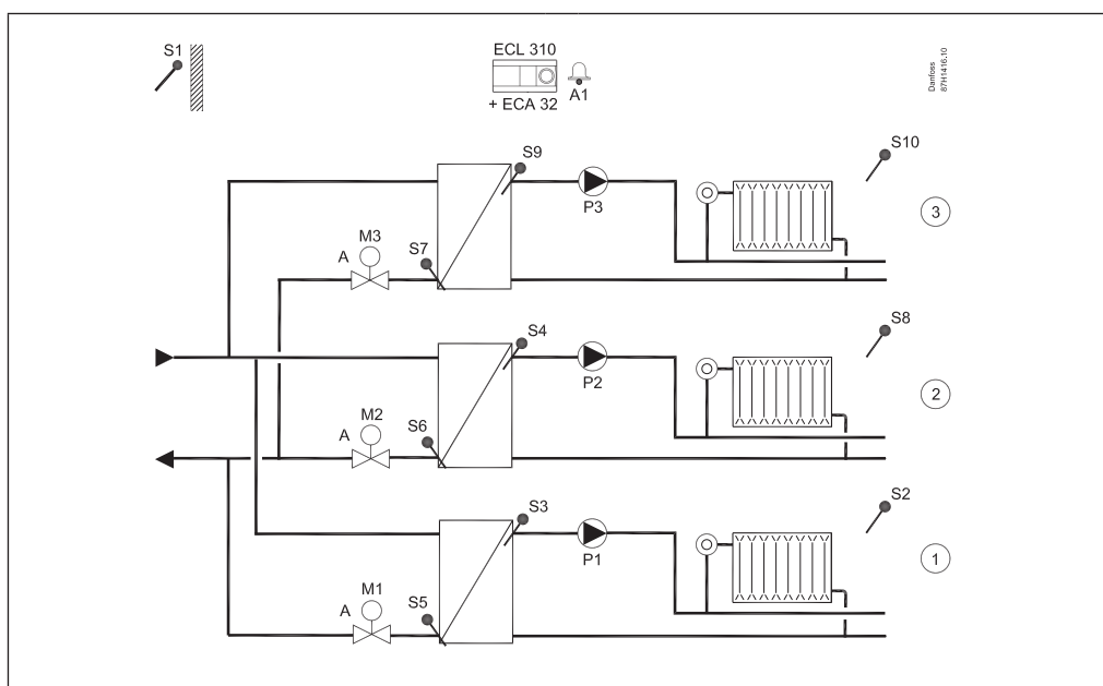
A390.2, näide a 3x sõltumatult ühendatud küttekontuuri. Reguleeriventiilide täiturmootoreid juhitakse 0–10 V signaalidega.
