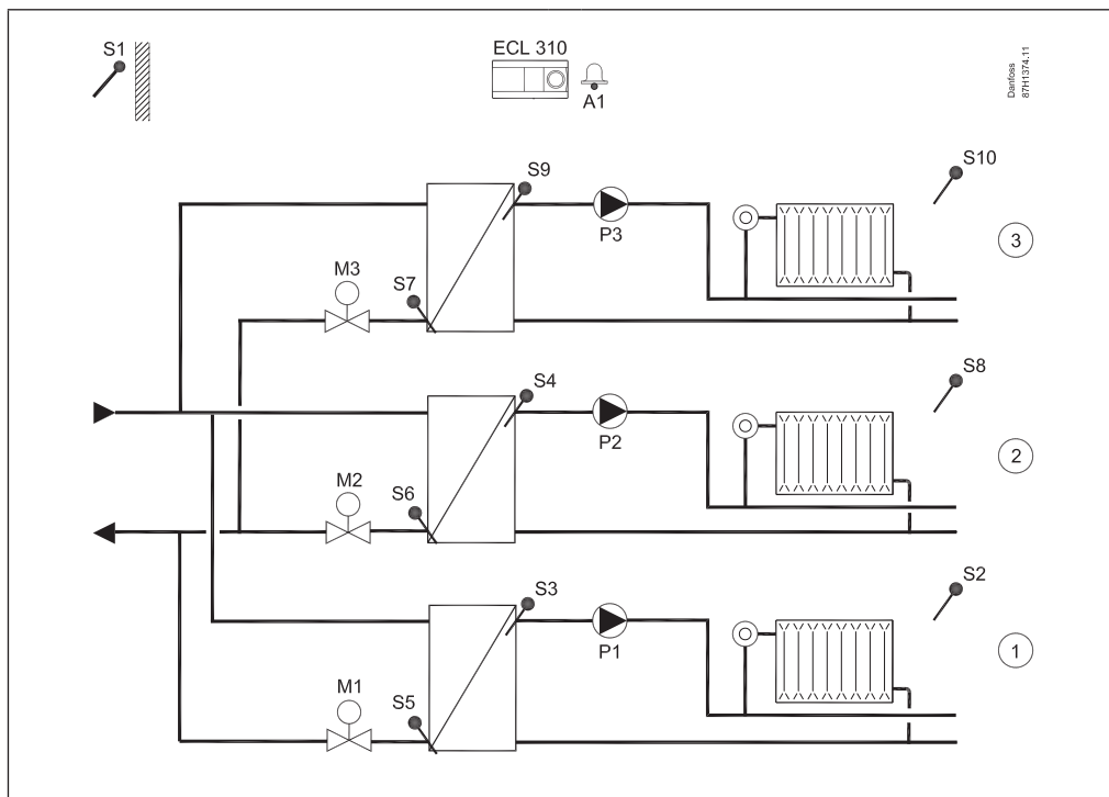
A390.2, näide a 3x sõltumatult ühendatud küttekontuuri. Reguleeriventiilide täiturmootoreid juhitakse 0–10 V signaalidega.
