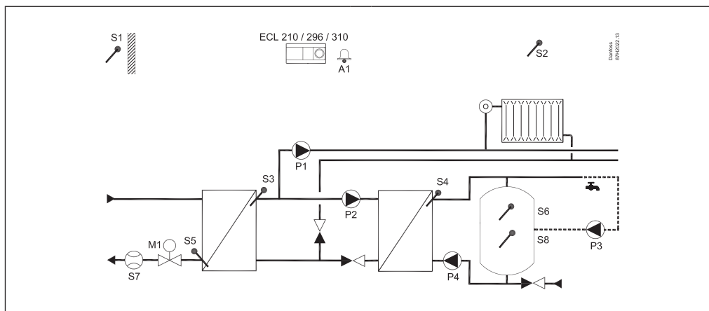
A247.1, näide a: Sõltumatult ühendatud kütte- ja STV paagi laadimise süsteem. Paralleelrežiim või STV eelistus
