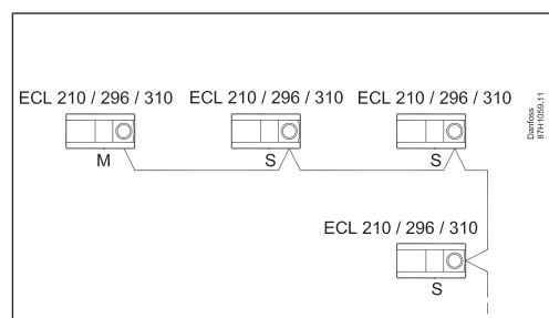
Raccordements maître/esclave
