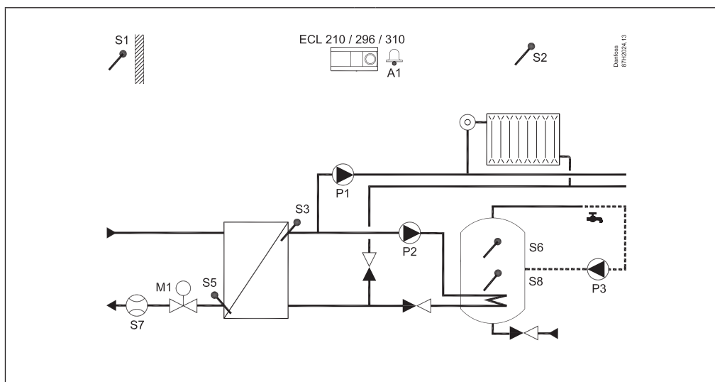
A237.2, ex. a : Système de chauffage et système de charge ECS raccordés indirectement
