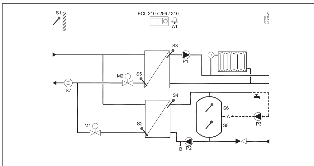
A247.1, ex. a : Systèmes de chauffage et de charge ECS raccordés indirectement (Mode parallèle ou priorité ECS)
