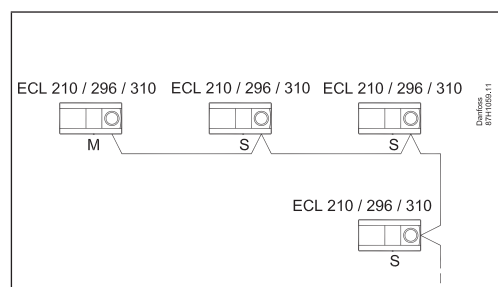
Raccordements maître/esclave
