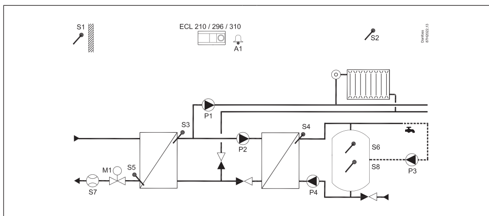
A247.1, ex. a : Systèmes de chauffage et de charge ECS raccordés indirectement (Mode parallèle ou priorité ECS)
