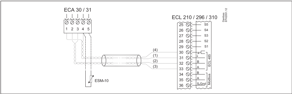
Câblage de l'ECL Comfort 310/310B et de l'ECA 30/31
