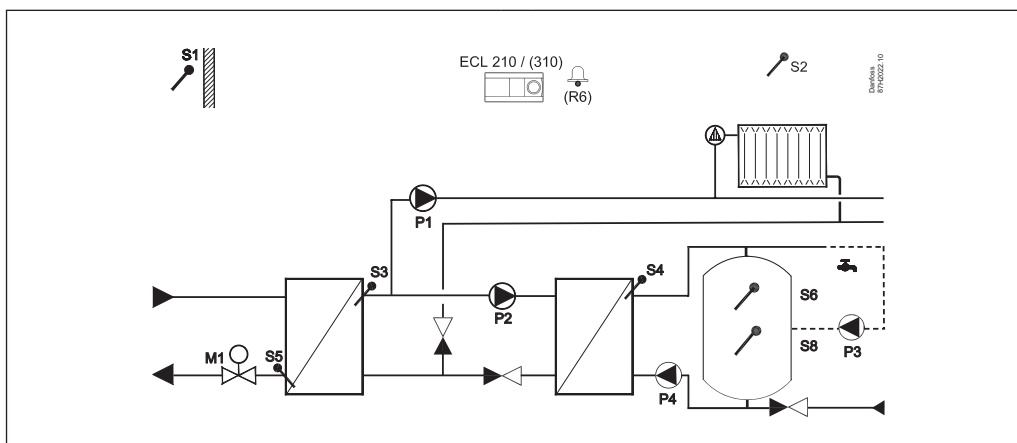
A247.1, ex. a : Systèmes de chauffage et de charge ECS raccordés indirectement (Mode parallèle ou priorité ECS)
