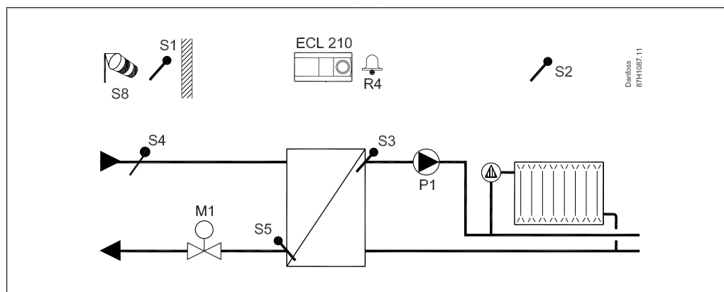
A230.1, ex. a : Système de chauffage raccordé indirectement. Compensation du vent en option
