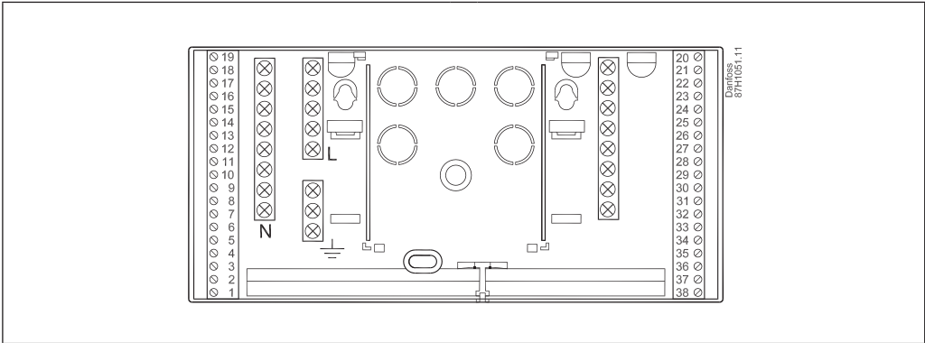
Socle ECL Comfort 310 (peut également être utilisée pour l'ECL Comfort 210).
