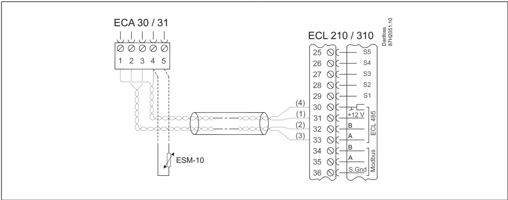
Câblage de l'ECL Comfort 310/310B et de l'ECA 30/31
