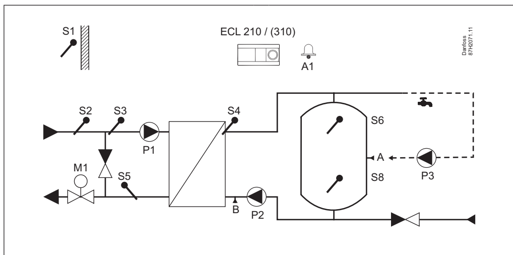
A217.2, ex. a : Charge du ballon ECS avec circuit de préchauffage
