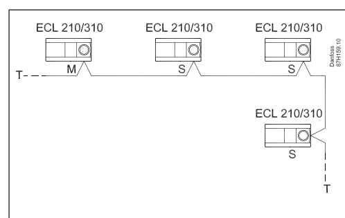
Raccordements maître/esclave
