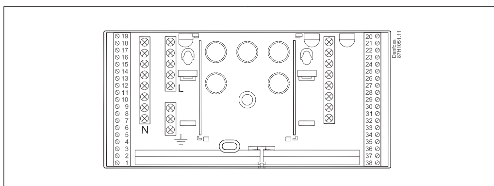
Podnožje za ECL Comfort 310 (može se upotrebljavati i za ECL Comfort 210).
