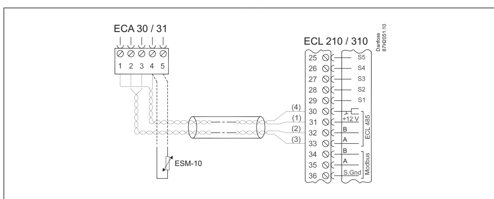
Ožičenje ECL Comfort 310/310B i ECA 30/31
