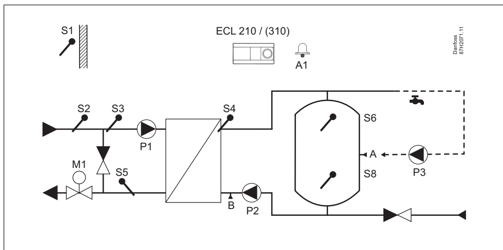
A217.2, primjer a: Nadopuna spremnika PTV-a s krugom za smanjivanje polazne temperature
