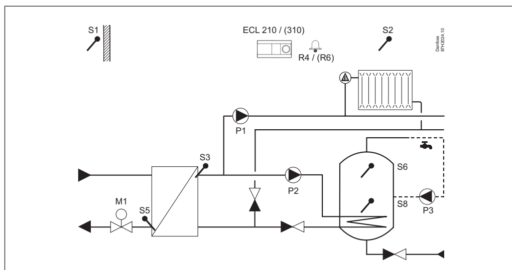
A237.1, primjer a: Neizravno spojen sustav grijanja i PTV-a
