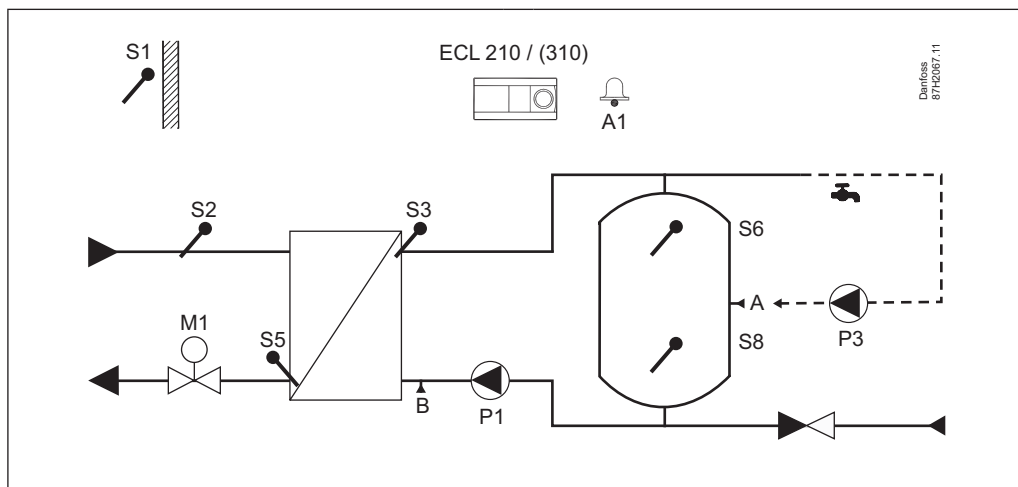
A217.1, primjer a: Aplikacija za nadopunu spremnika PTV-a
