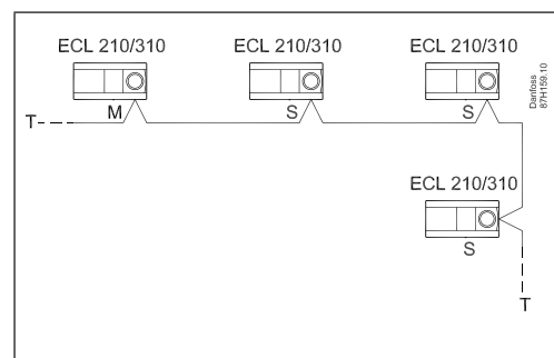
Spojevi glavni/podređeni
