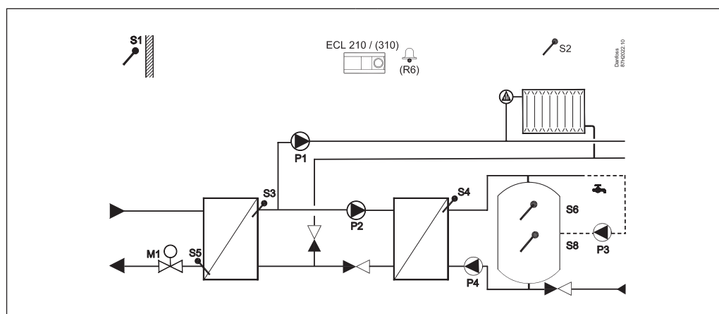
A247.1, primjer a: Neizravno spojen sustav grijanja i nadopune spremnika PTV-a Paralelan rad ili prioritet PTV-a
