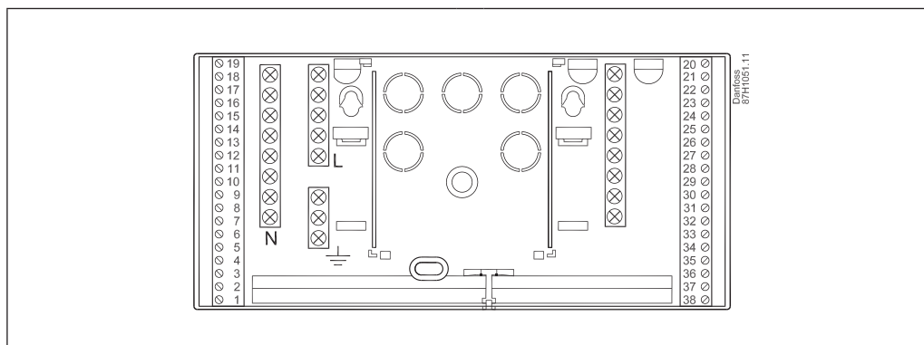
ECL Comfort 310 szerelőlap (az ECL Comfort 210-zel is használható).
