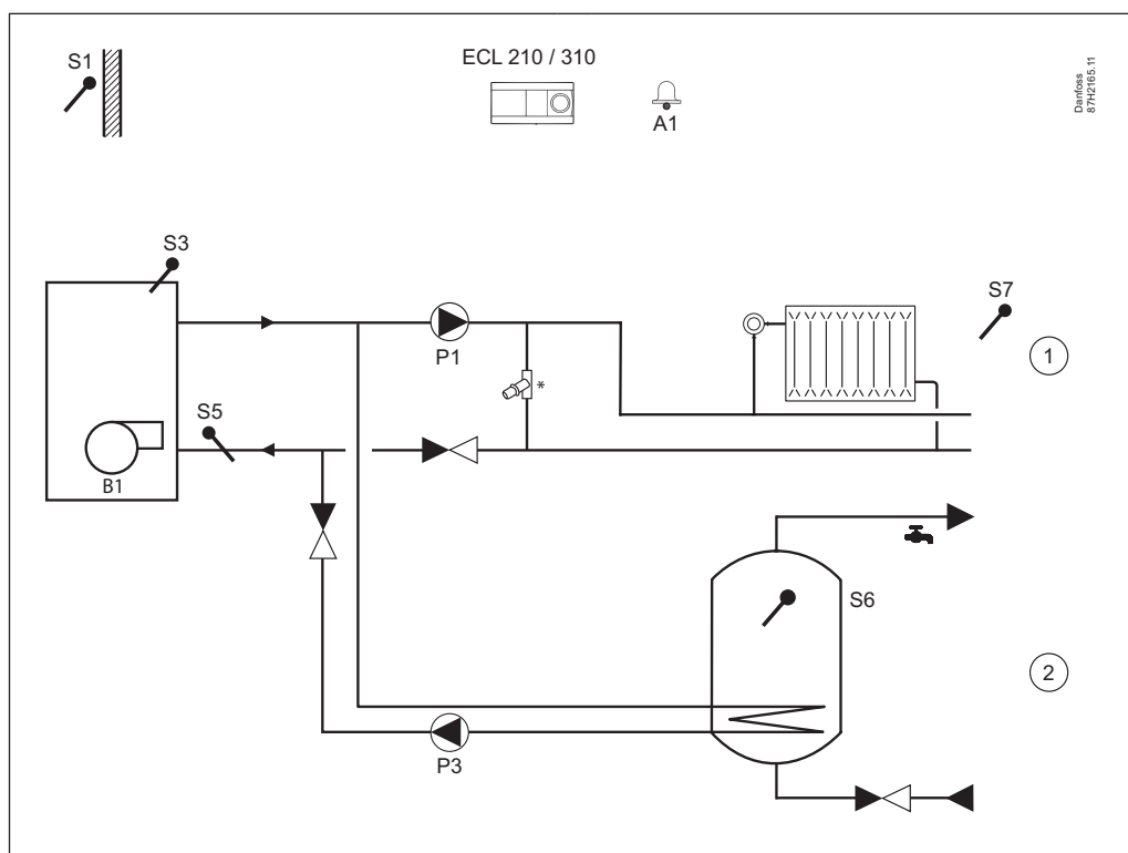
A275.2, es. a: Impianto di riscaldamento con caldaia mono-stadio e bollitore ACS
