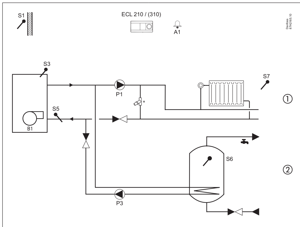
A275.3, ed. a: Impianto di riscaldamento con caldaia mono-stadio, circuito di miscelazione e bollitore ACS
