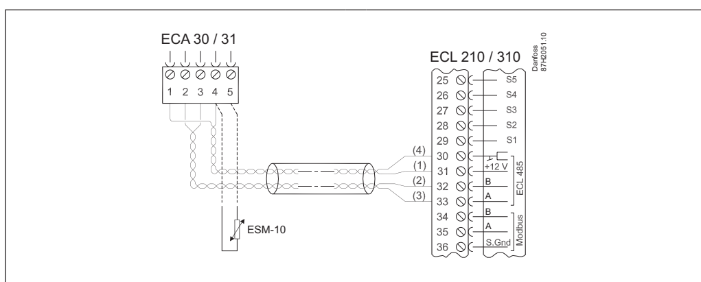
Cablaggio di ECL Comfort 310 / 310B ed ECA 30 / 31
