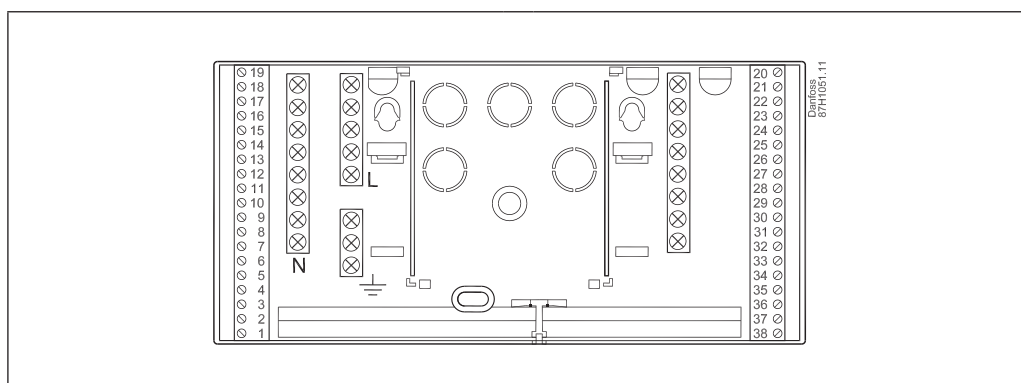
Base ECL Comfort 310 (può essere utilizzata anche per l'ECL Comfort 210).
