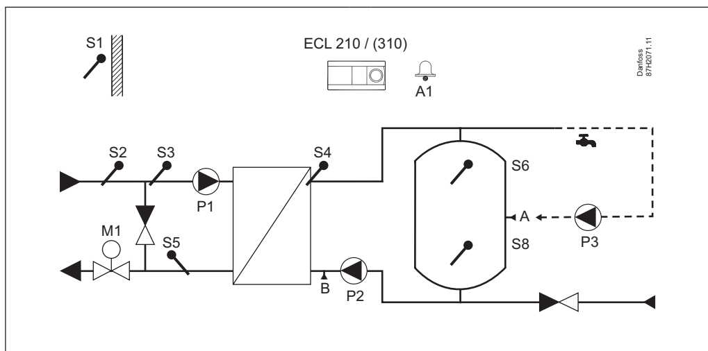
A217.2, es. a: Accumulo ACS con circuito di pre-riscaldamento
