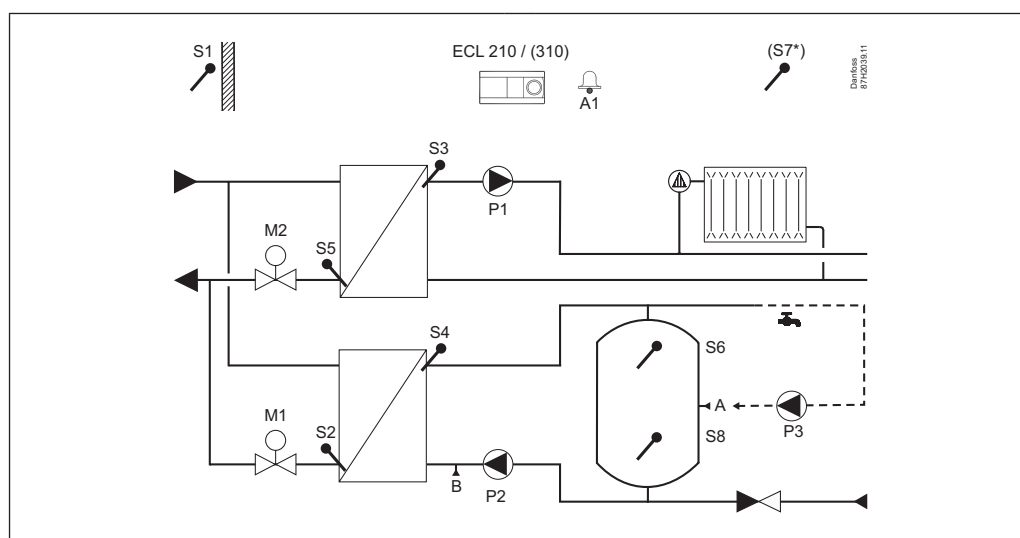
A247.1, es. a: Impianto di riscaldamento indiretto e sistema accumulo ACS Modalità parallela o priorità ACS
