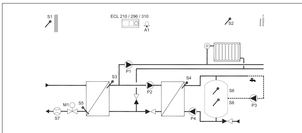
A247.1, es. a: Impianto di riscaldamento indiretto e sistema accumulo ACS Modalità parallela o priorità ACS
