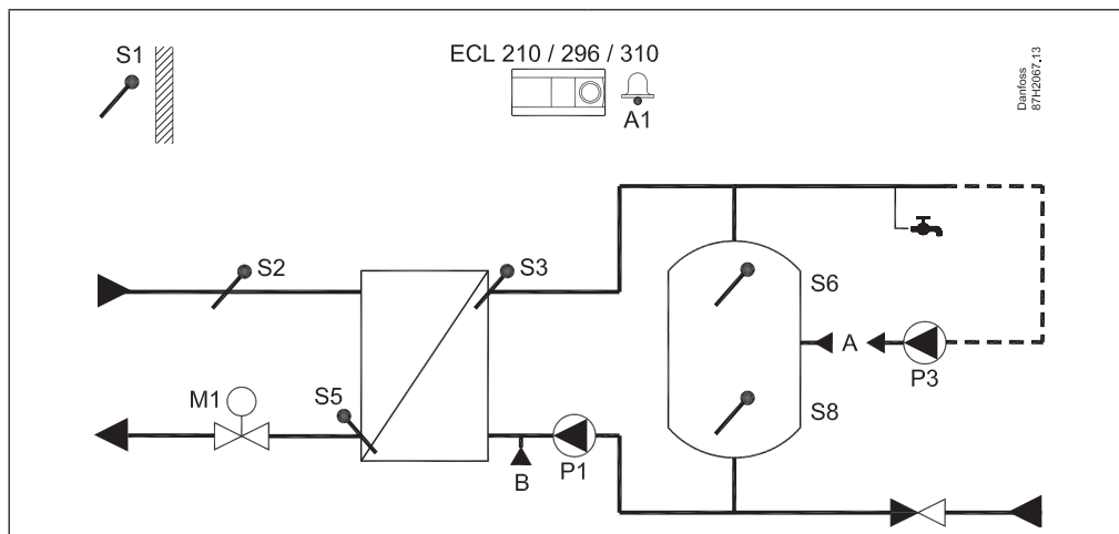
A217.1, es. b: Applicazione con bollitore ACS
