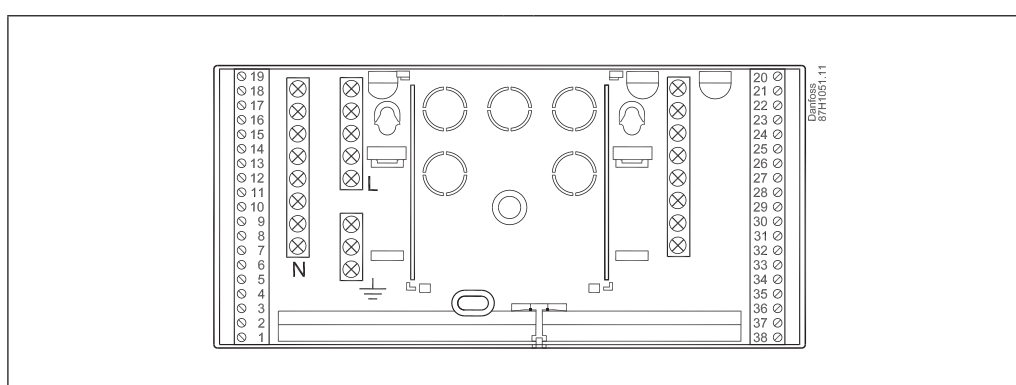
Unitatea de bază ECL Comfort 310 (poate fi utilizată și pentru ECL Comfort 210).
