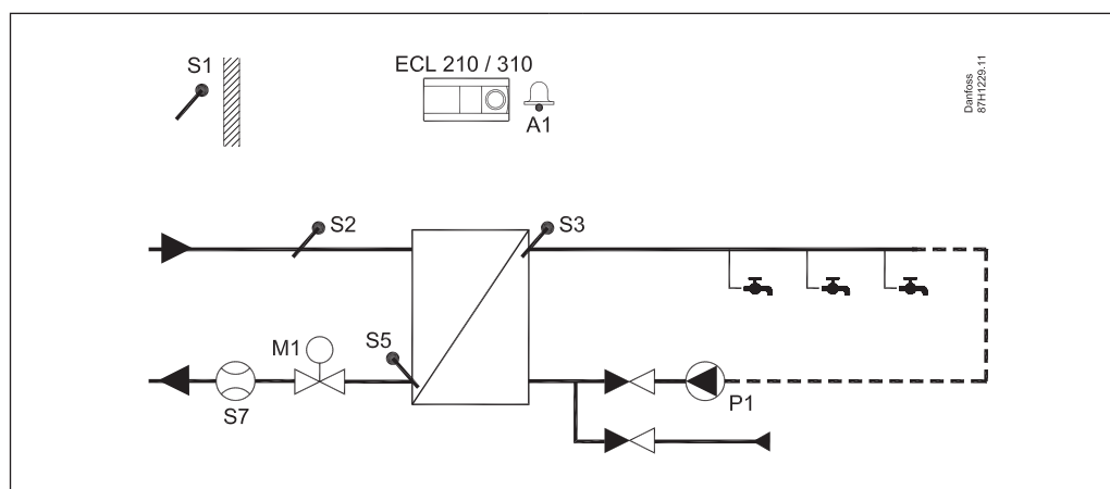
A217.3, przykład a: Aplikacja CWU w układzie przepływowym
