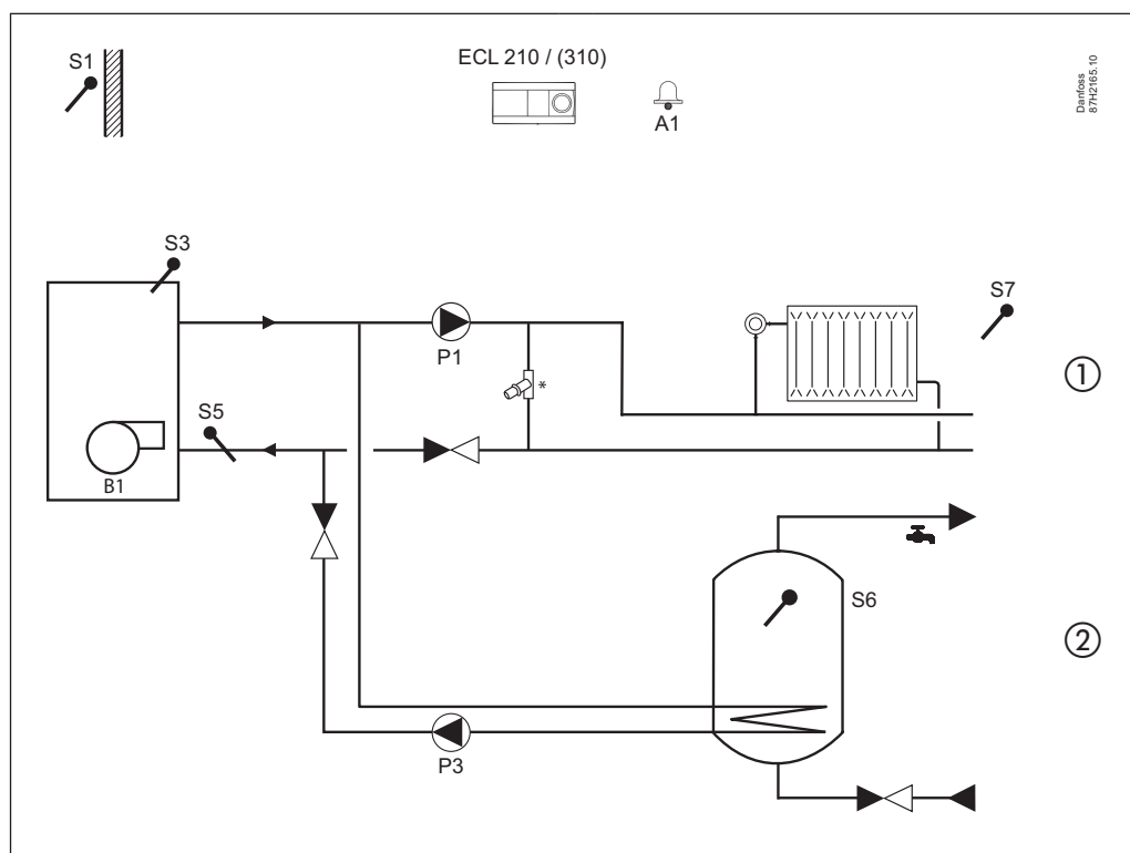
A275.2, przykład a: Układ ogrzewania z kotłem 1-stopniowym i wymiennikiem pojemnościowym CWU
