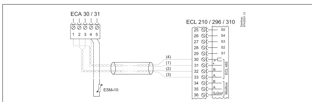
Схема электрических соединений ECL Comfort 310 / 310B и ECA 30 / 31
