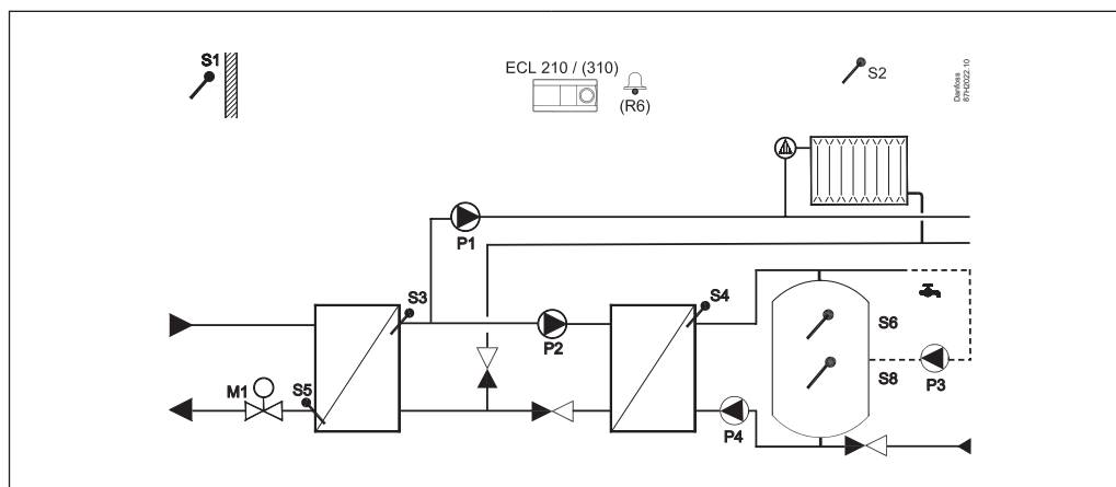
A247.1, príklad a: Nepriamo zapojený systém vykurovania a systém nabíjania zásobníka TUV. Paralelný režim alebo priorita TUV
