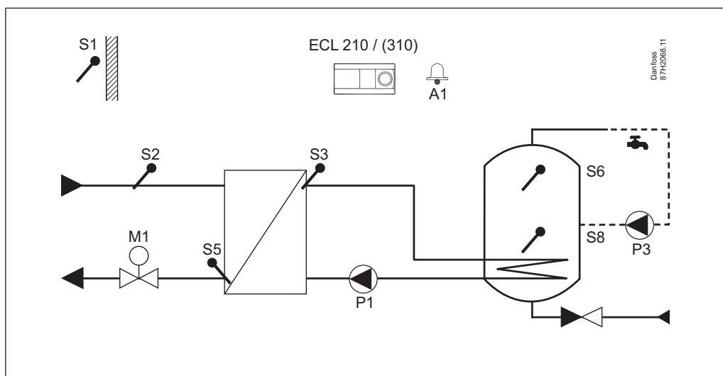
A217.1, príklad b: Aplikácia vykurovania zásobníka TUV
