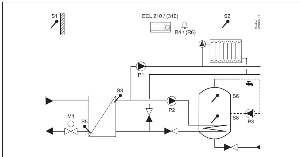
A237.2, príklad a: Nepriamo zapojený systém vykurovania a systém nabíjania TUV
