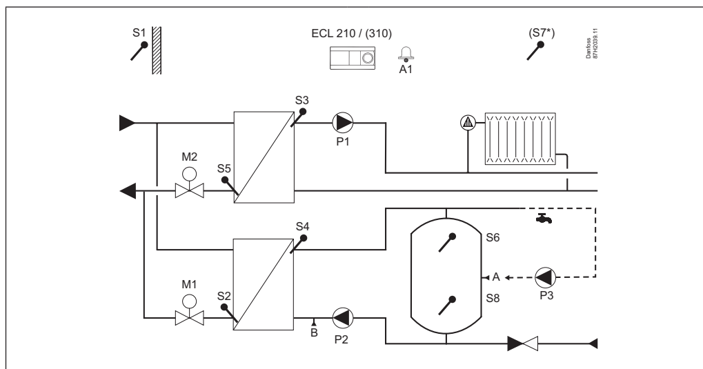
A247.1, príklad a: Nepriamo zapojený systém vykurovania a systém nabíjania zásobníka TUV. Paralelný režim alebo priorita TUV
