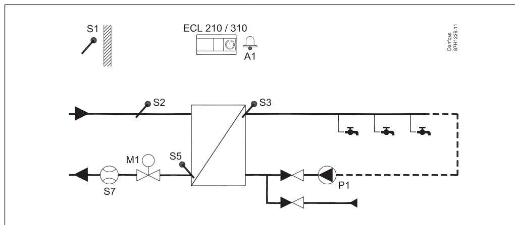
A217.3, príklad c: Príprava TÚV na požiadanie (spínač prietoku). S alebo bez cirkulácie
