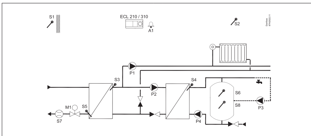
A247.1, príklad a: Nepriamo zapojený systém vykurovania a systém nabíjania zásobníka TÚV. Paralelný režim alebo priorita TÚV
