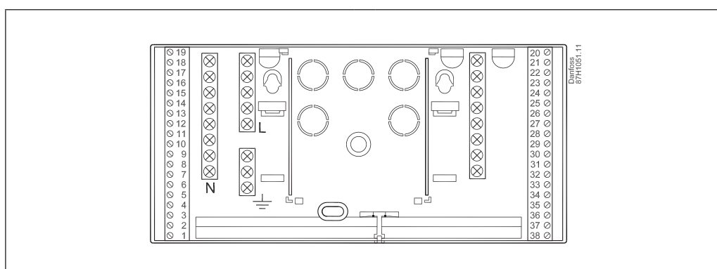
ECL Comfort 310 podnožje (može da se koristi i za ECL Comfort 210).
