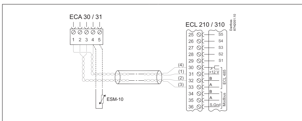
Ožičenje za ECL Comfort 310/310B i ECA 30/31
