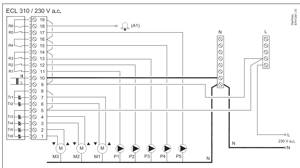
Príklad zapojenia regulátora ECL Comfort 310
