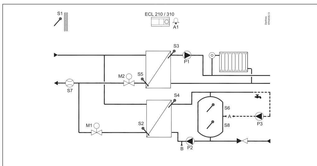
A247.1, exempel a: Indirekt anslutet värme- och laddningssystem för varmvattentank. Parallelläge eller varmvattentprioritet
