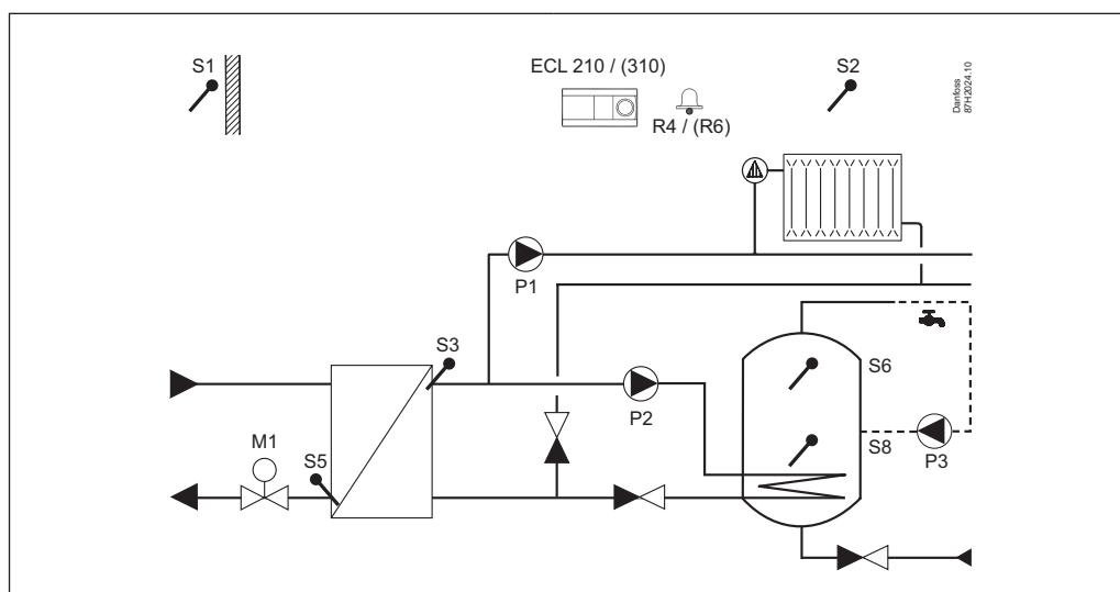
A237.1, exempel a: Indirekt anslutet värme- och varmvattensystem
