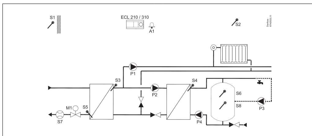
A247.1, exempel a: Indirekt anslutet värme- och laddningssystem för varmvattentank. Parallelläge eller varmvattentprioritet
