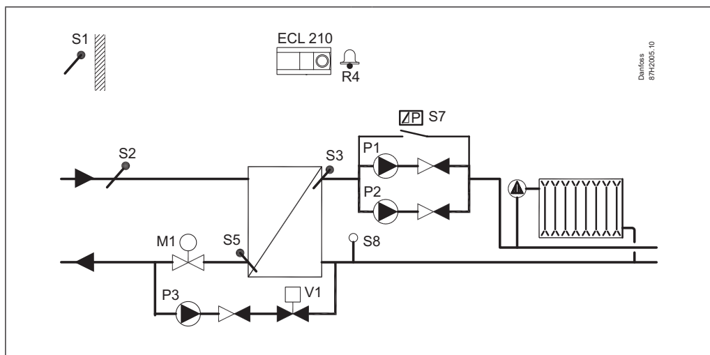
A331.2, exempel a: Värmesystem med 2-pumpsreglering och vattenpåfyllningsfunktion. Flödestemperaturreglering beroende av inloppstemperaturen.
