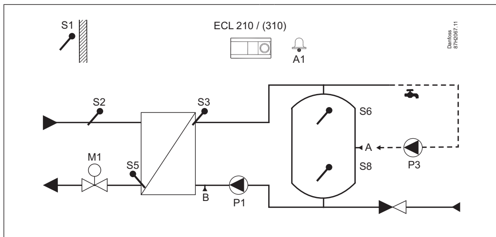
A217.1, exempel a: Tillämpning för laddning av varmvattentank
