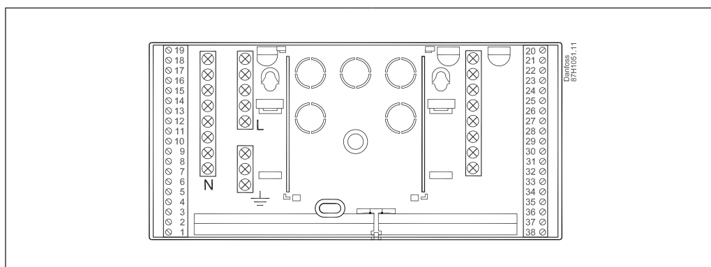
ECL Comfort 310 underdel (kan även användas för ECL Comfort 210).
