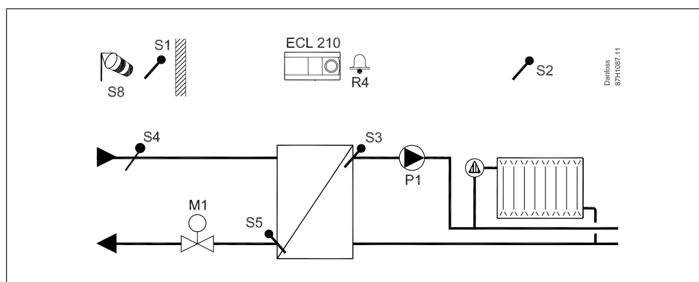
A230.1, exempel a: Indirekt anslutet värmesystem. Vindkompensering som tillval
