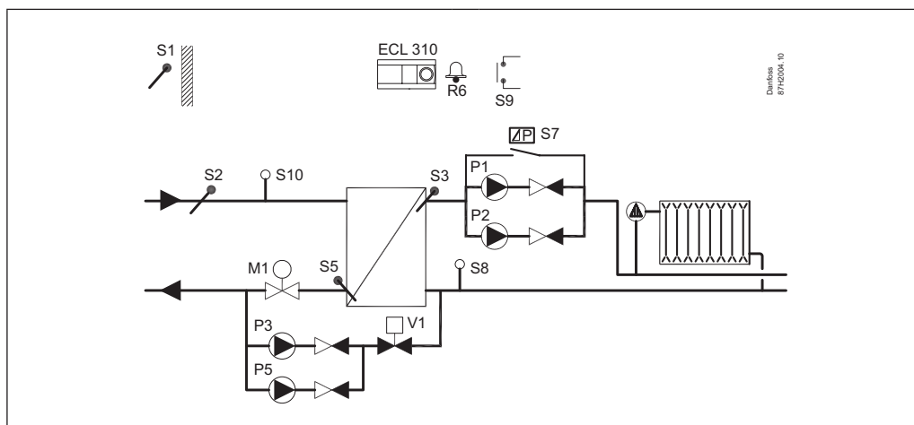
A331.2, exempel a: Värmesystem med 2-pumpsreglering och vattenpåfyllningsfunktion. Flödestemperaturreglering beroende av inloppstemperaturen.
