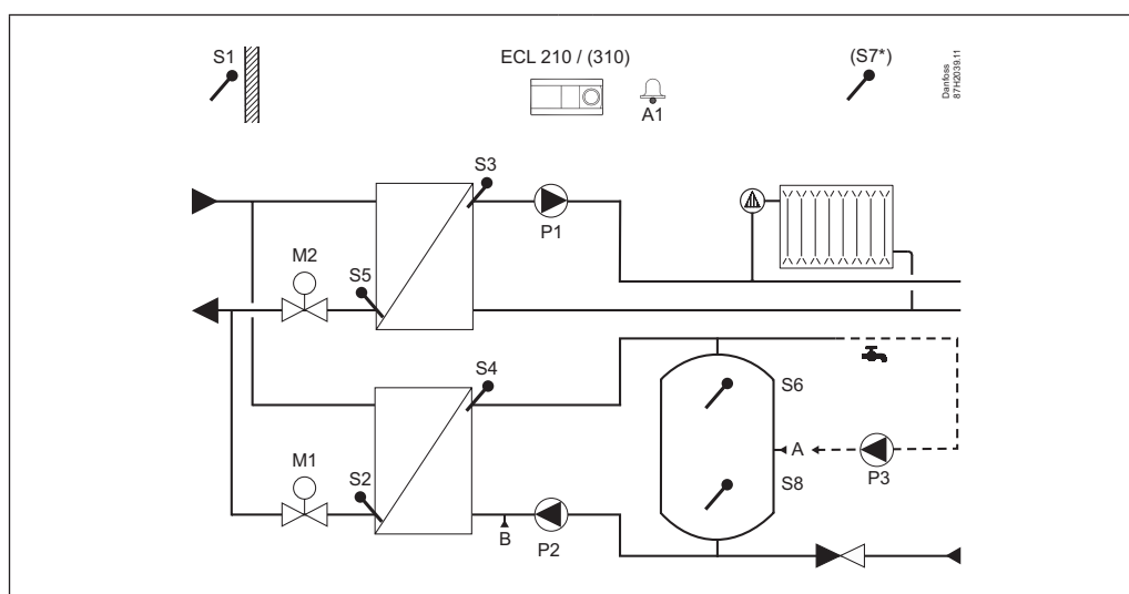
A247.1, exempel a: Indirekt anslutet värme- och laddningssystem för varmvattentank. Parallelläge eller varmvattentankprioritet
