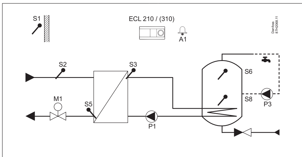
A217.1, exempel b: Tillämpning för uppvärmning av varmvattentank
