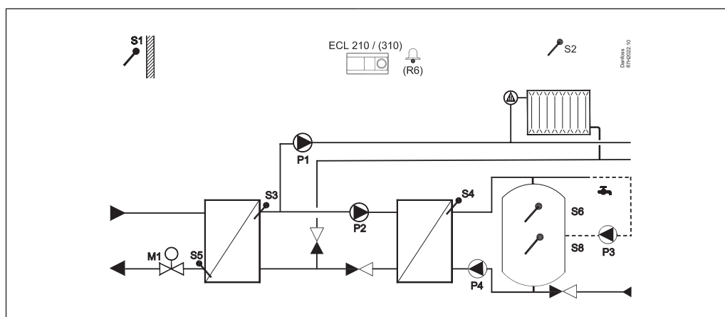
A247.1, exempel a: Indirekt anslutet värme- och laddningssystem för varmvattentank. Parallelläge eller varmvattentankprioritet
