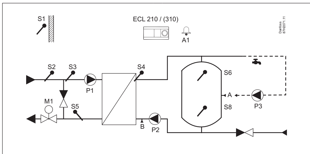
A217.2, exempel a: Laddning av varmvattentank med förvärmningskrets
