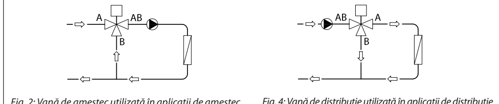
Fig. 2: Vană de amestec utilizată în aplicații de amestec
