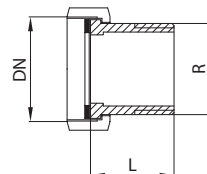
Anschraubenden (Außengewinde)
