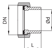
Anschweißenden
