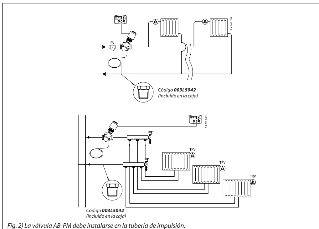
Fig. 2) La válvula AB-PM debe instalarse en la tubería de impulsión.
