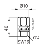
Łącznik kombinacyjny KF2, KF3 Złączka zaciskowa
