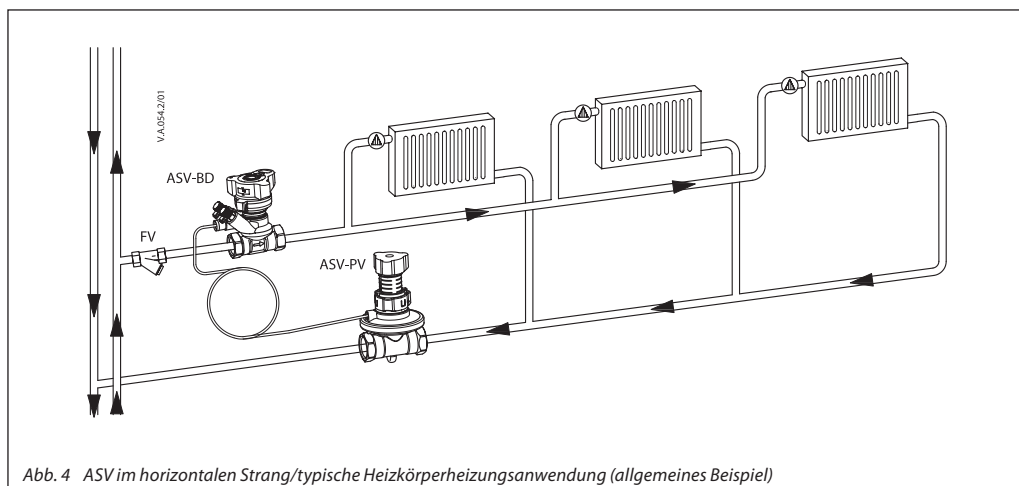
Abb. 4 ASV im horizontalen Strang/typische Heizkörperheizungsanwendung (allgemeines Beispiel)
