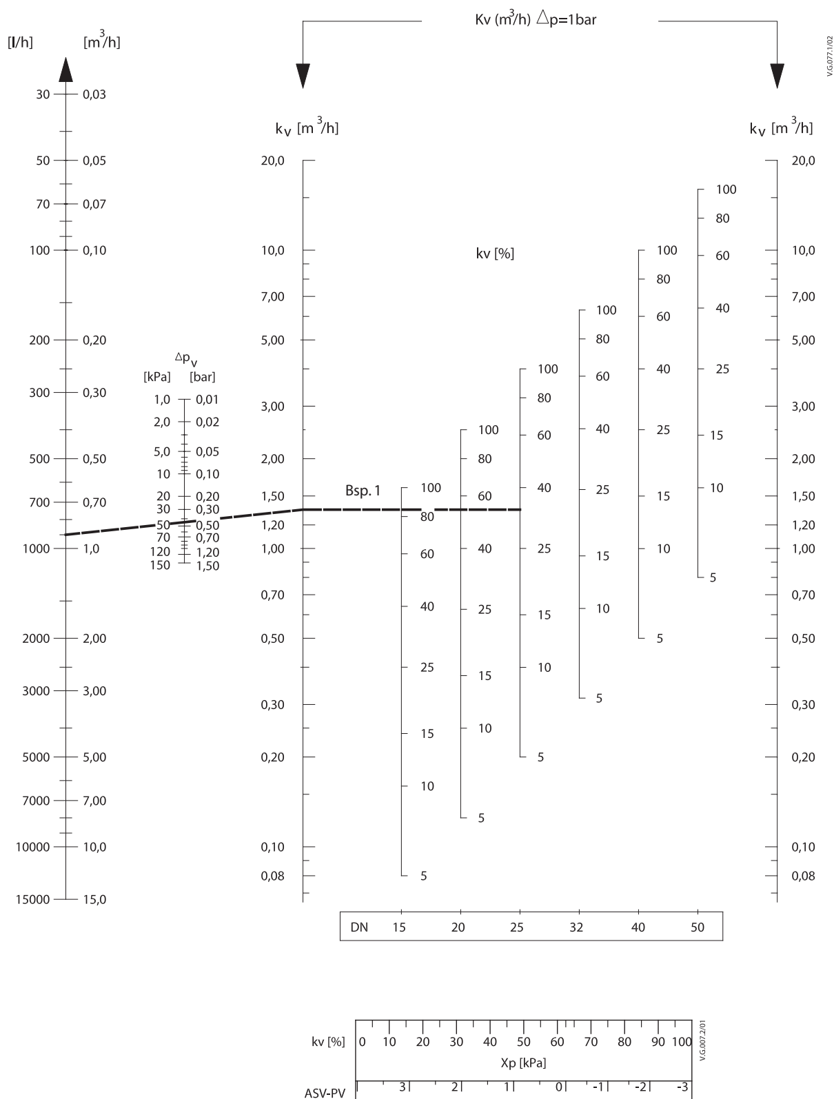
Abb. A – Auslegungsdiagramm für ASV-PV, DN 15-50
