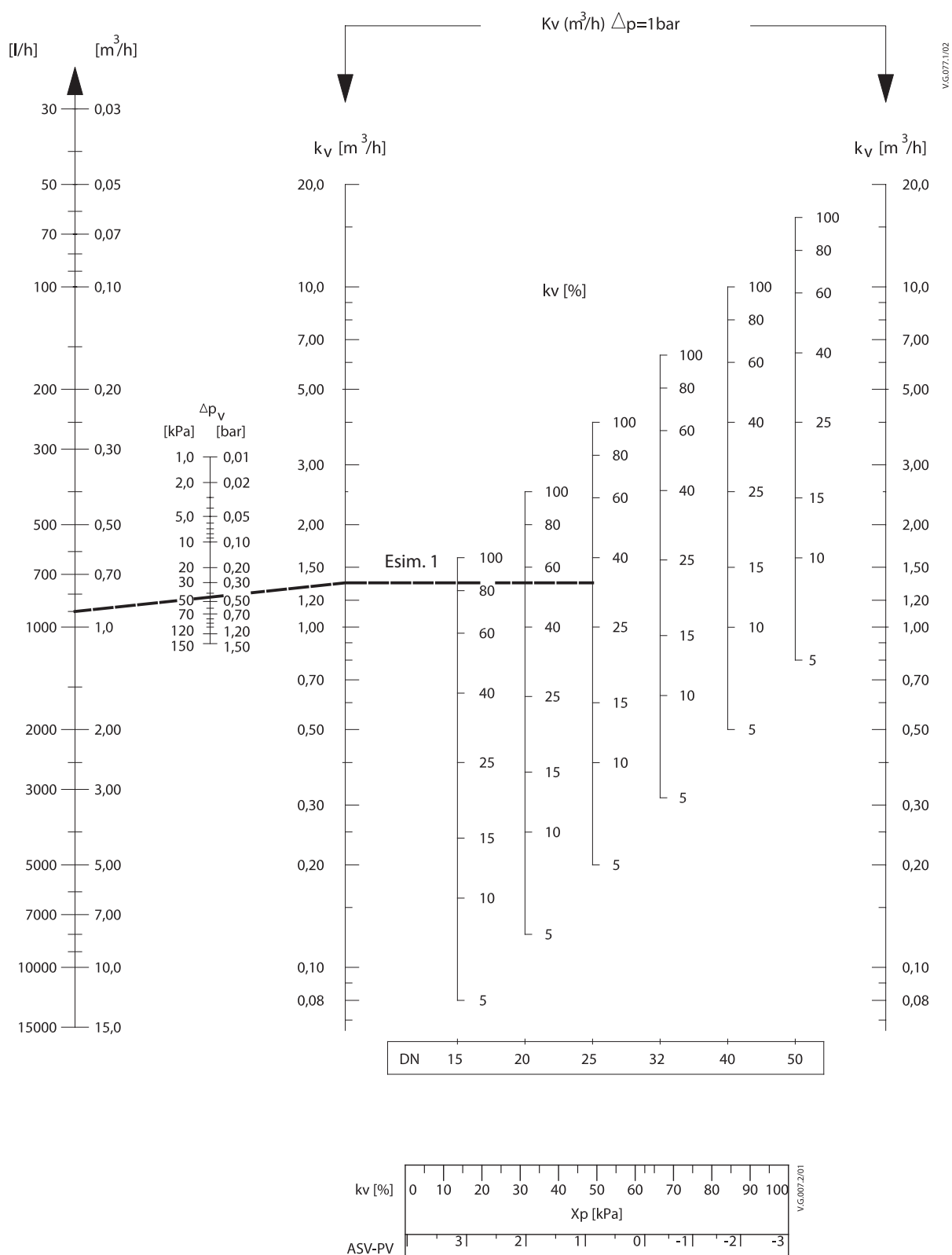
Kuva A - Mitoituskuvaaja ASV-PV DN 15-50
