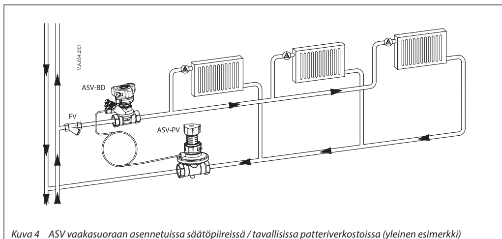
Kuva 4 ASV vaakasuoraan asennetuissa säätöpiireissä / tavallisissa patteriverkostoissa (yleinen esimerkki)
