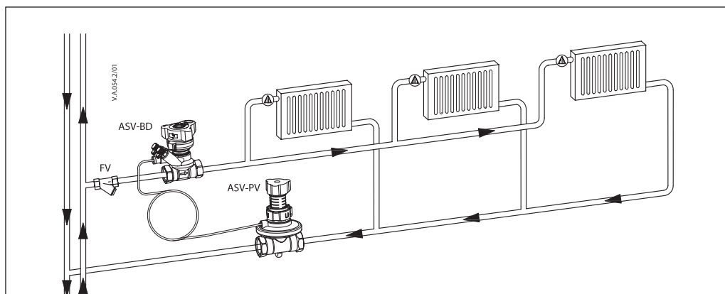
Fig. 4 Vanne ASV dans une boucle horizontale/application typique de chauffage par radiateur (exemple général)
