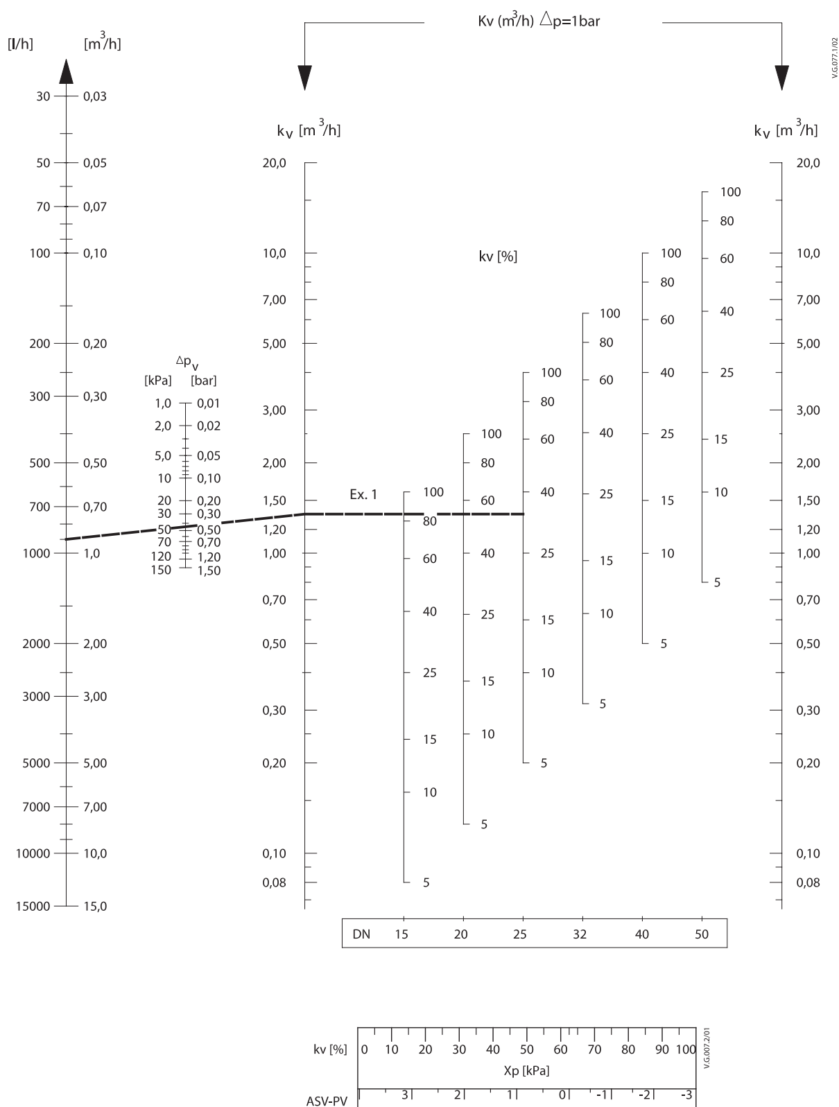
Fig. A - Diagramme de dimensionnement ASV-P/PV DN 15-50
