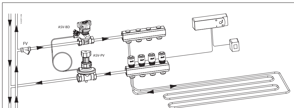
Fig. 5 ASV dans le distributeur d'un système de plancher chauffant
