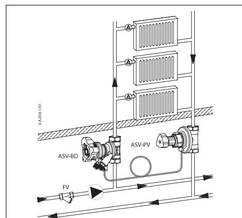
Fig. 3 ASV în coloană ascendentă verticală/aplicație de încălzire cu radiator tipică (exemplu general)
