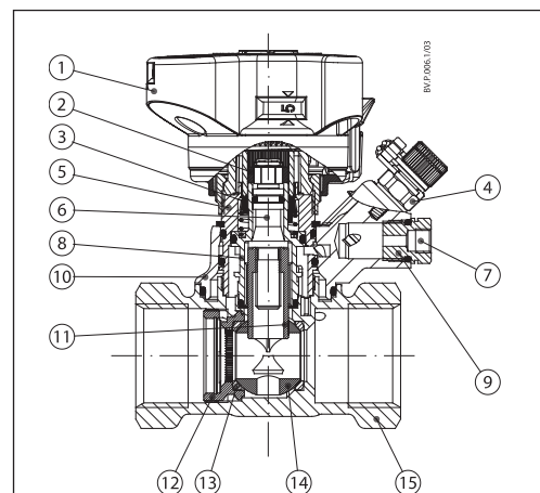
Rys. 7 ASV-BD DN 15-50
