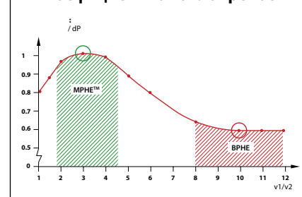
Топлообменници MicroPlate™
