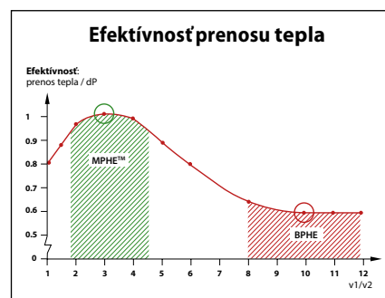
Tepelné výmenníky MicroPlate™
