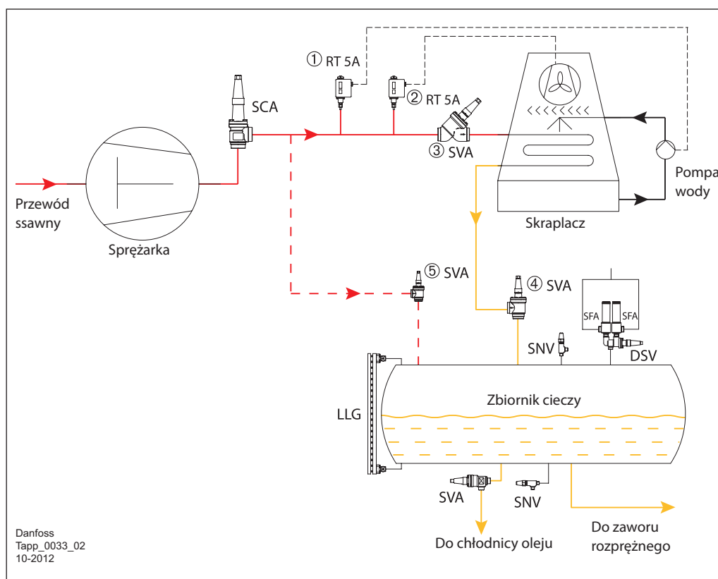
Przykład zastosowania 3.2.1: Regulacja wielostopniowa z wykorzystaniem presostatów RT
