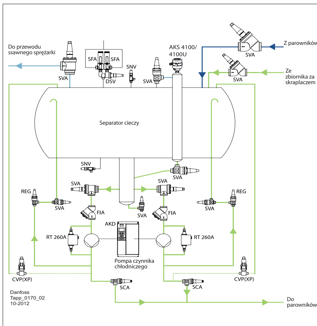
Rysunek 11.4 — Pompy cyrkulacyjne CO 2 z przetwornicą AKD i wymaganymi zaworami oraz regulatorami
