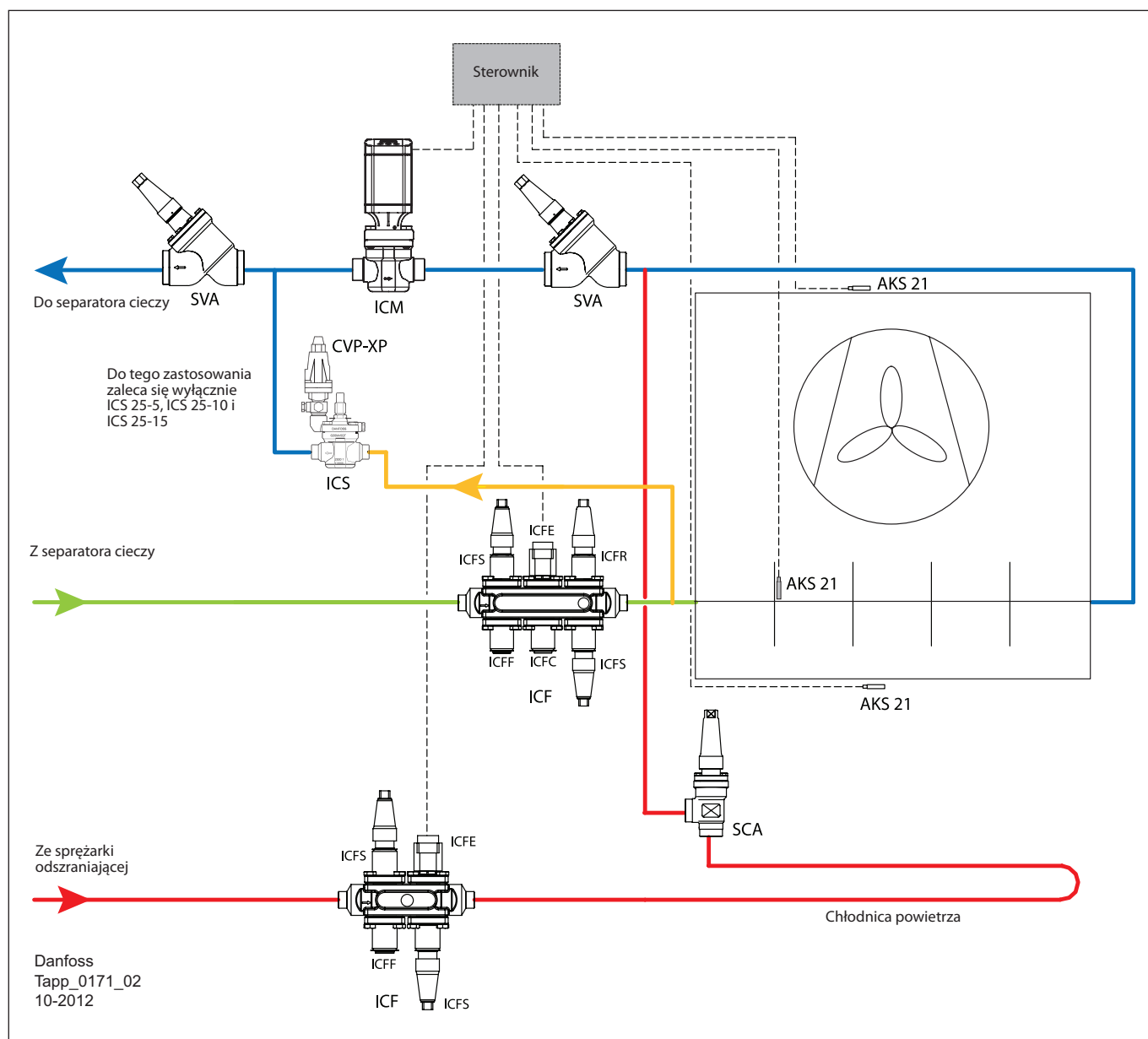
Rysunek 11.5 — Odszranianie gorącym gazem CO 2
