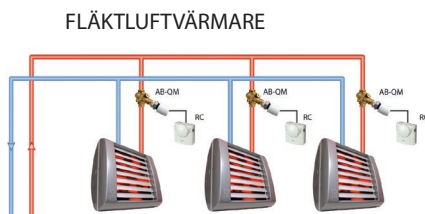
FLÄKTLUFTVÄRMARE
