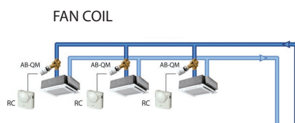
FAN COIL
