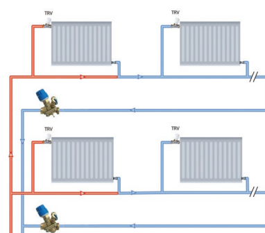
1-RÖRSSYSTEM
