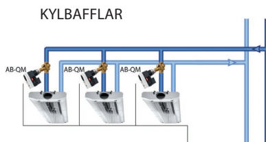
KYLBAFFLAR
