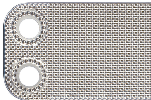
Теплообменная пластина Micro Plate™ для паяного теплообменника
