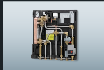
Stanovanjska postaja talnega ogrevanja s pretočnim ogrevanjem sanitarne tople vode
