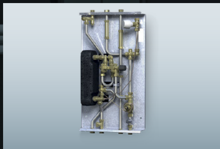
Stanovanjske postaje za zamenjavo starih plinskih kotlov
