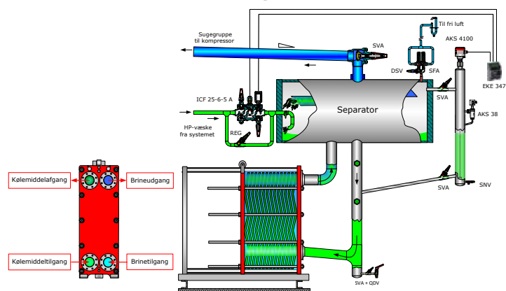
Oversvømmet fordamper (Køling af brine)
