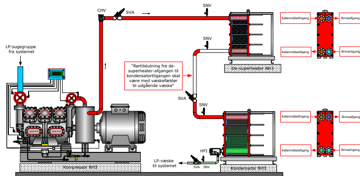
Væskeafkølede kondensatorer (Opvarming af brine)
