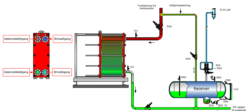
Væskeafkølet overhedningsfjerner (Opvarming af brine)
