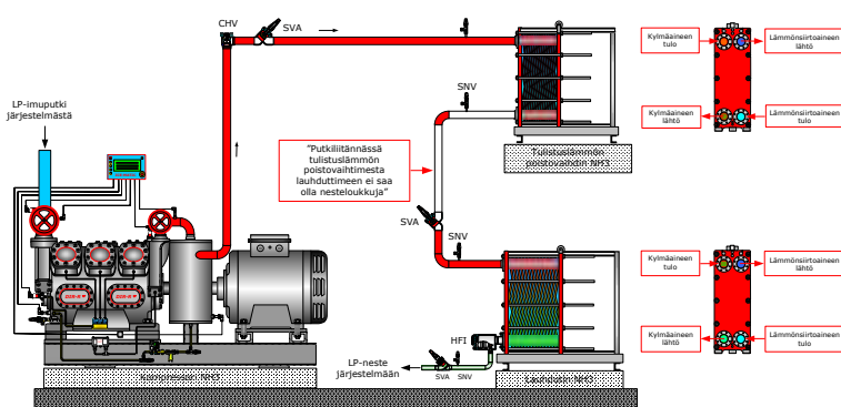
Nestejäähdytteiset lauhduttimet (lämmönsiirtoaineen lämmittäminen)
