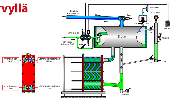
Märkähöyrystin (lämmönsiirtoaineen jäähdytys)
