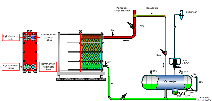
Nestejäähdytteiset tulistuslämmön poistovaihtimet (lämmönsiirtoaineen lämmittäminen)
